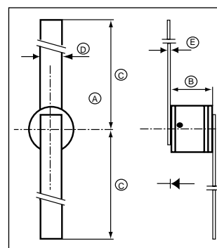
M208e C_b=0.12pF
